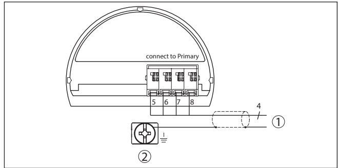
Fig. 3: Esquema de conexiones VEGABAR 83 dispositivo secundario
