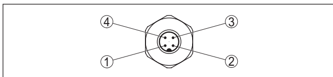
Fig. 14: Vue sur le connecteur M12 x 1
