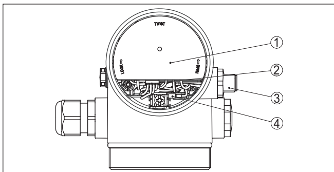
Fig. 13: Vue sur le compartiment de l'électronique avec l'adaptateur VEGADIS pour le raccordement de l'unité de réglage et d'affichage
