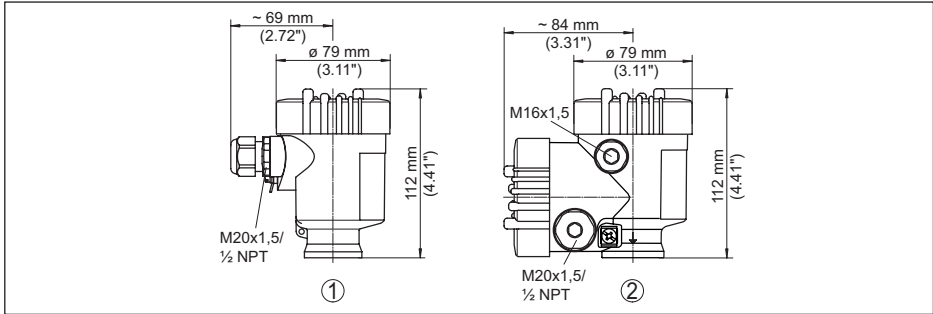
Fig. 35: Variantes de boîtier en protection IP66/IP67 (avec un module de réglage et d'affichage intégré, la hauteur du boîtier augmente de 9 mm/0.35 in)
