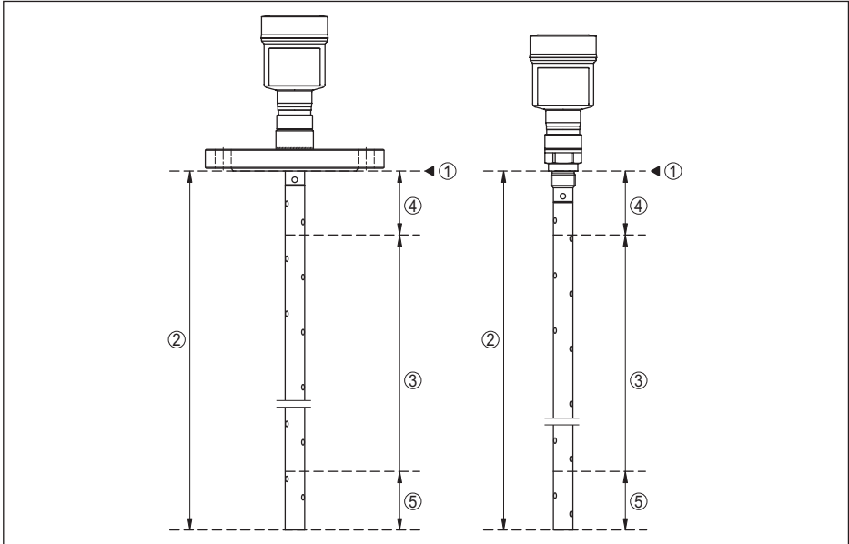
Fig. 30: Plages de mesure - VEGAFLEX 81
