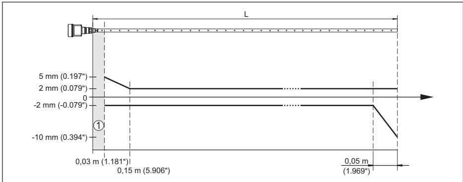
Fig. 31: Écart de mesure VEGAFLEX 81 en version coaxiale dans le produit Eau
