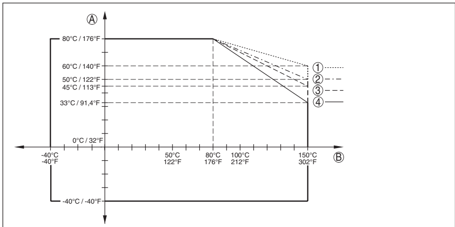
Fig. 33: Température ambiante - température process, version standard
