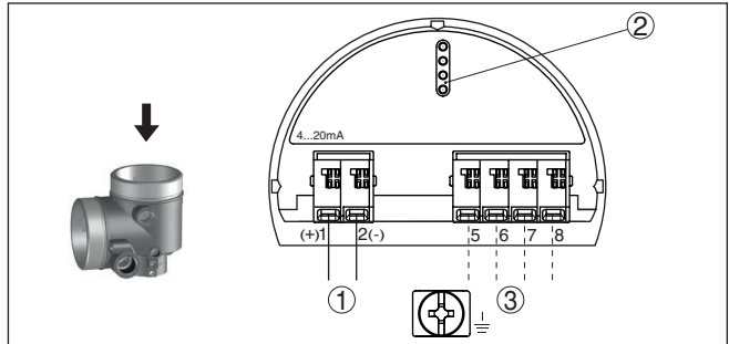
Fig. 11: Compartiment électronique - boîtier à deux chambres Ex d ia
