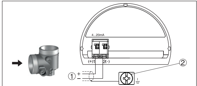
Fig. 12: Compartiment de raccordement - Boîtier à deux chambres Ex d ia
