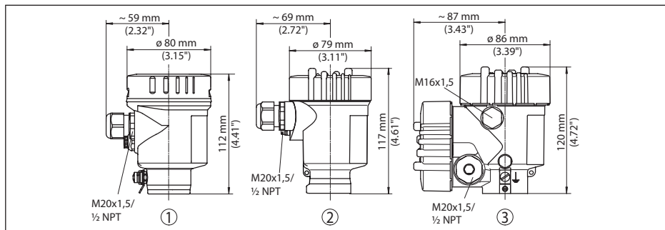
Fig. 38: Variantes de boîtier en protection IP66/IP68 (0,2 bar), (avec un module de réglage et d'affichage intégré, la hauteur du boîtier augmente de 9 mm/0.35 in)
