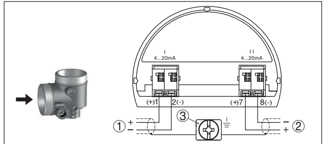
Fig. 16: Compartiment de raccordement boîtier à deux chambres, électronique supplémentaire "sortie courant supplémentaire"
