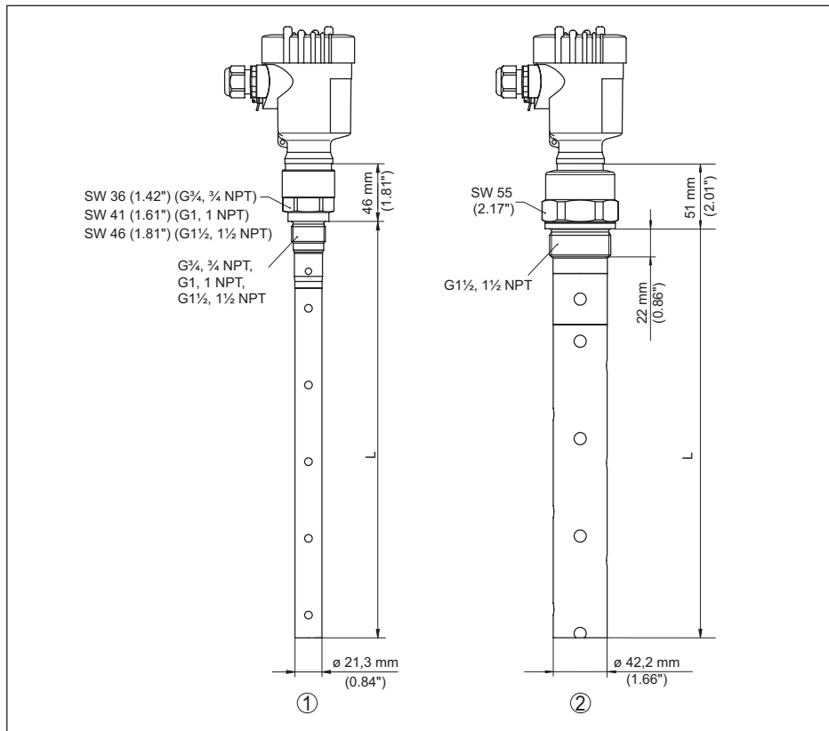
Fig. 40: VEGAFLEX 81, version fileté
