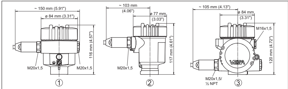
Fig. 39: Variantes de boîtier en protection IP66/IP68 (1 bar), (avec un module de réglage et d'affichage intégré, la hauteur du boîtier augmente de 9 mm/0.35 in)
