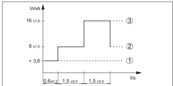
Fig. 12: Verloopdiagram functietest
