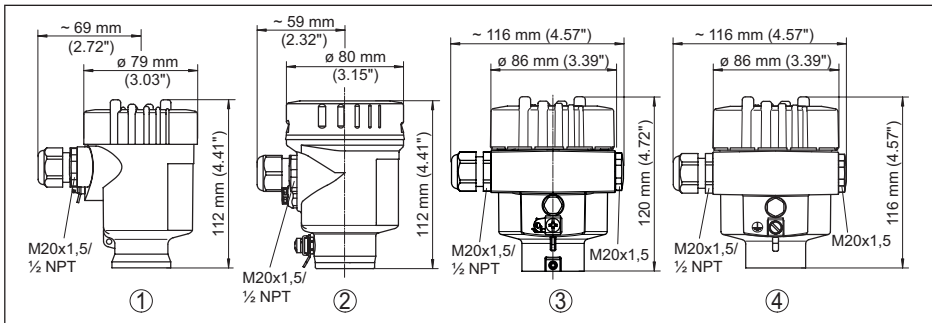
Fig. 19: Behuizingsuitvoeringen in beschermingsklasse IP66/IP67 en IP66/IP68 (0,2 bar)
