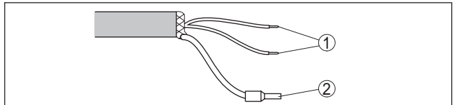
Fig. 10: Aderbezetting aansluitkabel
