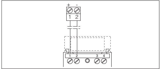
Fig. 9: Aansluitschema eenkamerbehuizing
