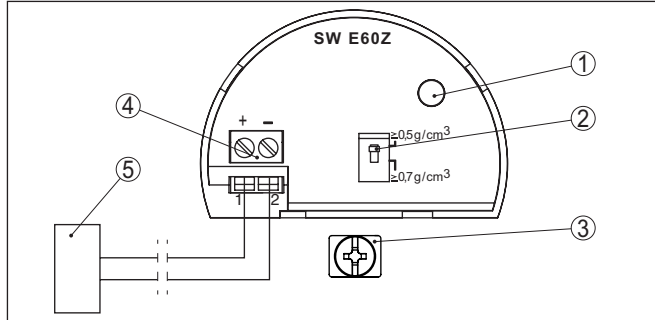
Fig. 8: Elektronica- en aansluitruimte
