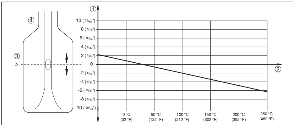
Fig. 12: Invloed procestemperatuur op het schakelpunt
