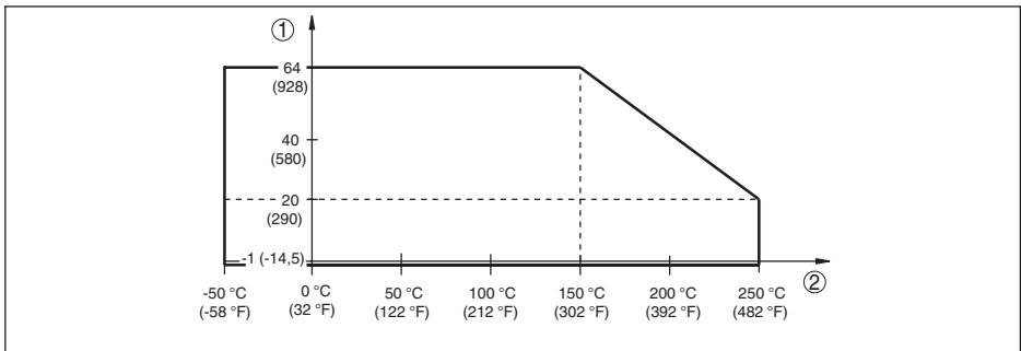
Fig. 17: Procestemperatuur - procesdruk bij schakelaarstand \geq 0,5 \text{ g/cm}^3 (gevoeligheidsschakelaar)
