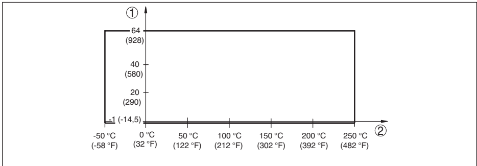
Fig. 16: Procestemperatuur - procesdruk bij schakelaarstand \geq 0,7 \text{ g/cm}^3 (gevoeligheidsschakelaar)
