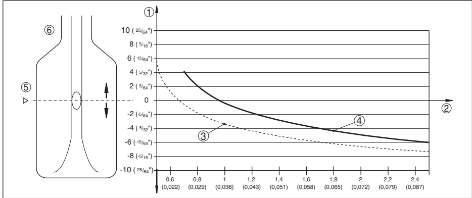
Fig. 13: Invloed van de stortgoedichtheid op het schakelpunt
